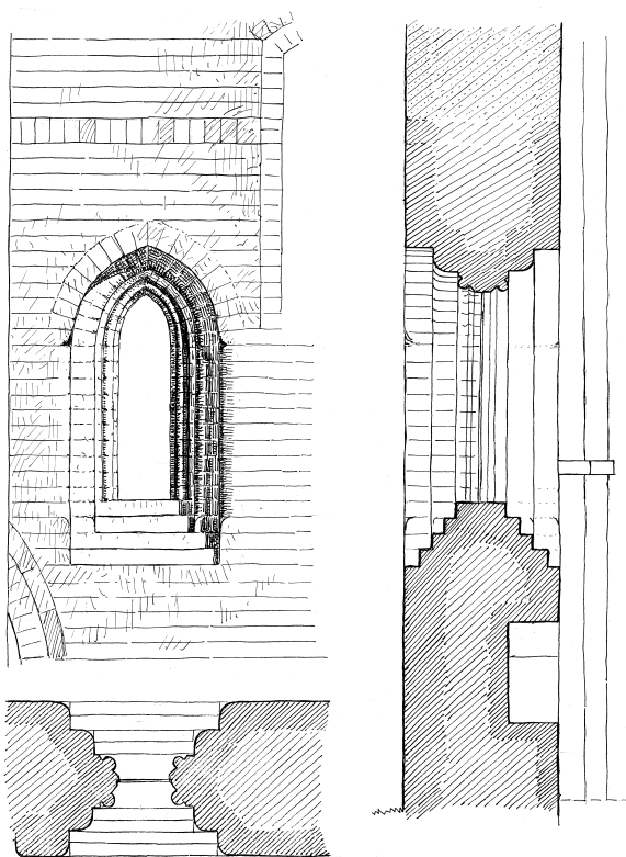
Fig. 9. Plan, opstalt og snit af oprindeligt vindue i korets sydside (s. 1038). 1:50. Målt og tegnet af Charles Christensen 1933. – Grundriss, Aufriss und Schnitt von ursprünglichem Fenster in der Südseite des Chores .
