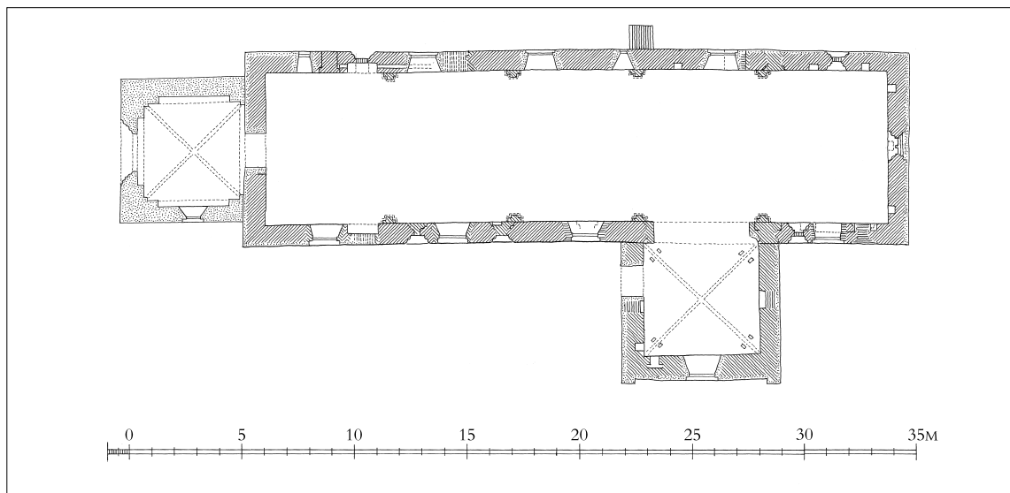
Fig. 8. Plan 1:300. Målt af Poul Hansen og Ib Lydholm 1964, suppleret 1966 af Morten Aaman Sørensen samt suppleret og tegnet af Hugo Johannsen 2010. – Grundriss .
