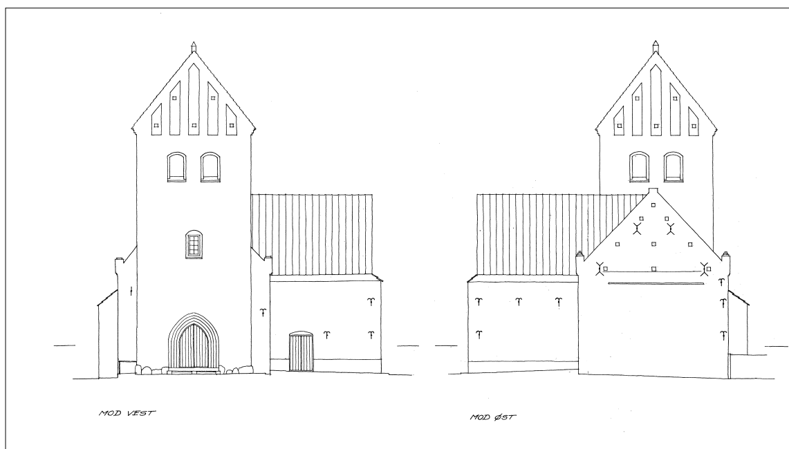
Fig. 13a-b. Facader. 1:300. Målt og tegnet af Poul Hansen og Ib Lydholm 1964. – Fassaden.
