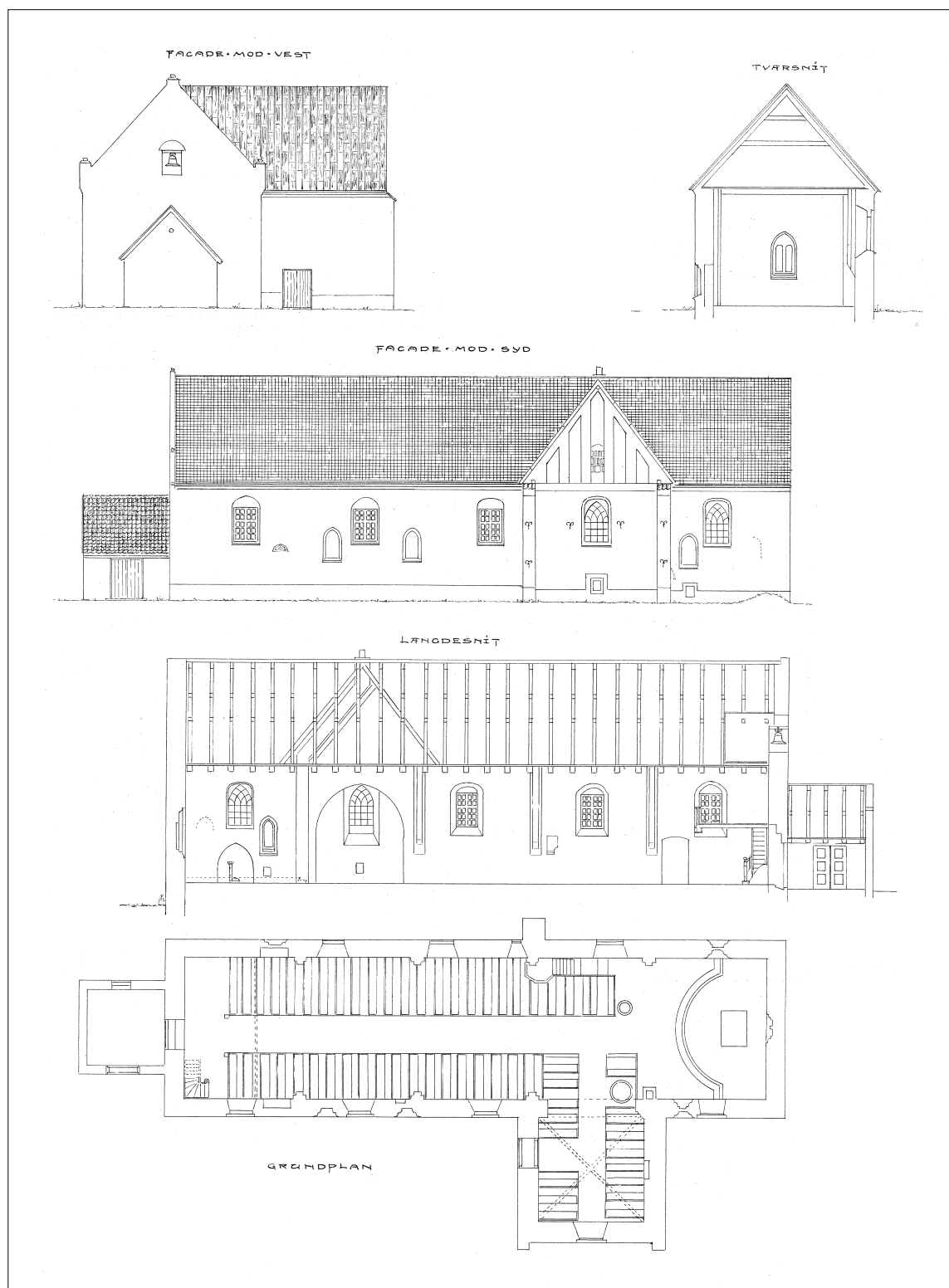
Fig. 11. Plan, snit og facader. 1:300. Målt og tegnet af Kristian Jensen 1928. – Grundriss, Schnitte und Fassade.
