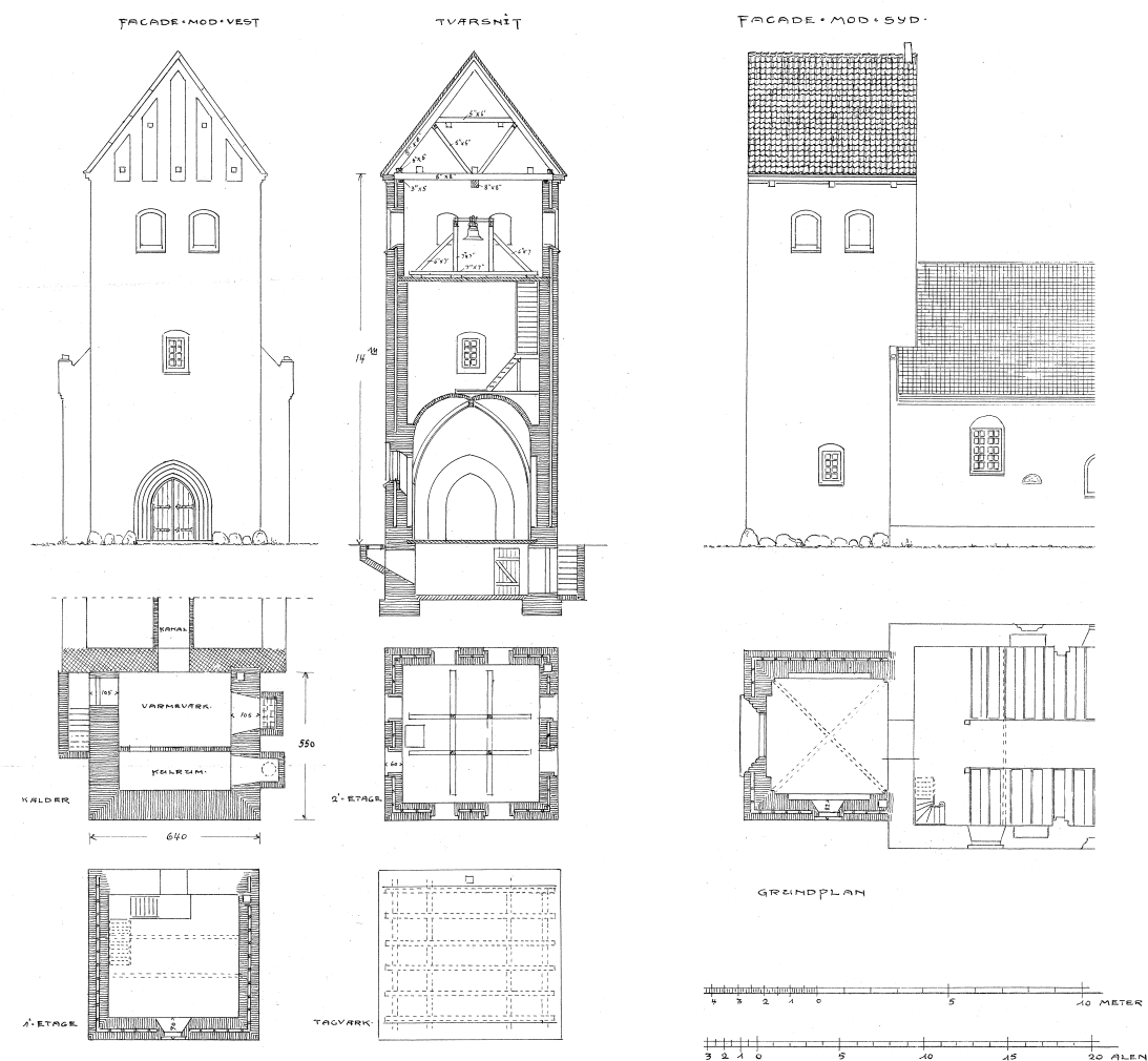
Fig. 25. Planer, facader og snit til projekteret tårn (s. 1044). 1:300. Kristian Jensen 1928. – Grundrisse, Fassaden und Schnitte über dem projektierten Turm.
