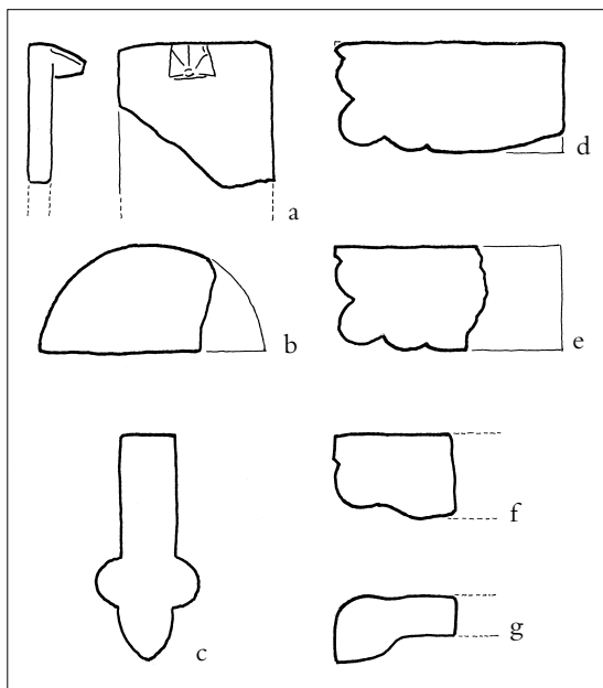
Fig. 29a-g. ★Tagpande og ★formsten af tegl fra †nonnekloster (s. 1051). a. Tagpande. b. Halvsøjle. c. Hvælveribbe. d.-g. Profilsten fra muråbninger (døre eller vinduer). 1:10. Målt af Hemming Klokke og tegnet af Hugo Johannsen 2010. Lemvig Museum. – ★ Dachpfanne und Formsteine aus Ziegel .
