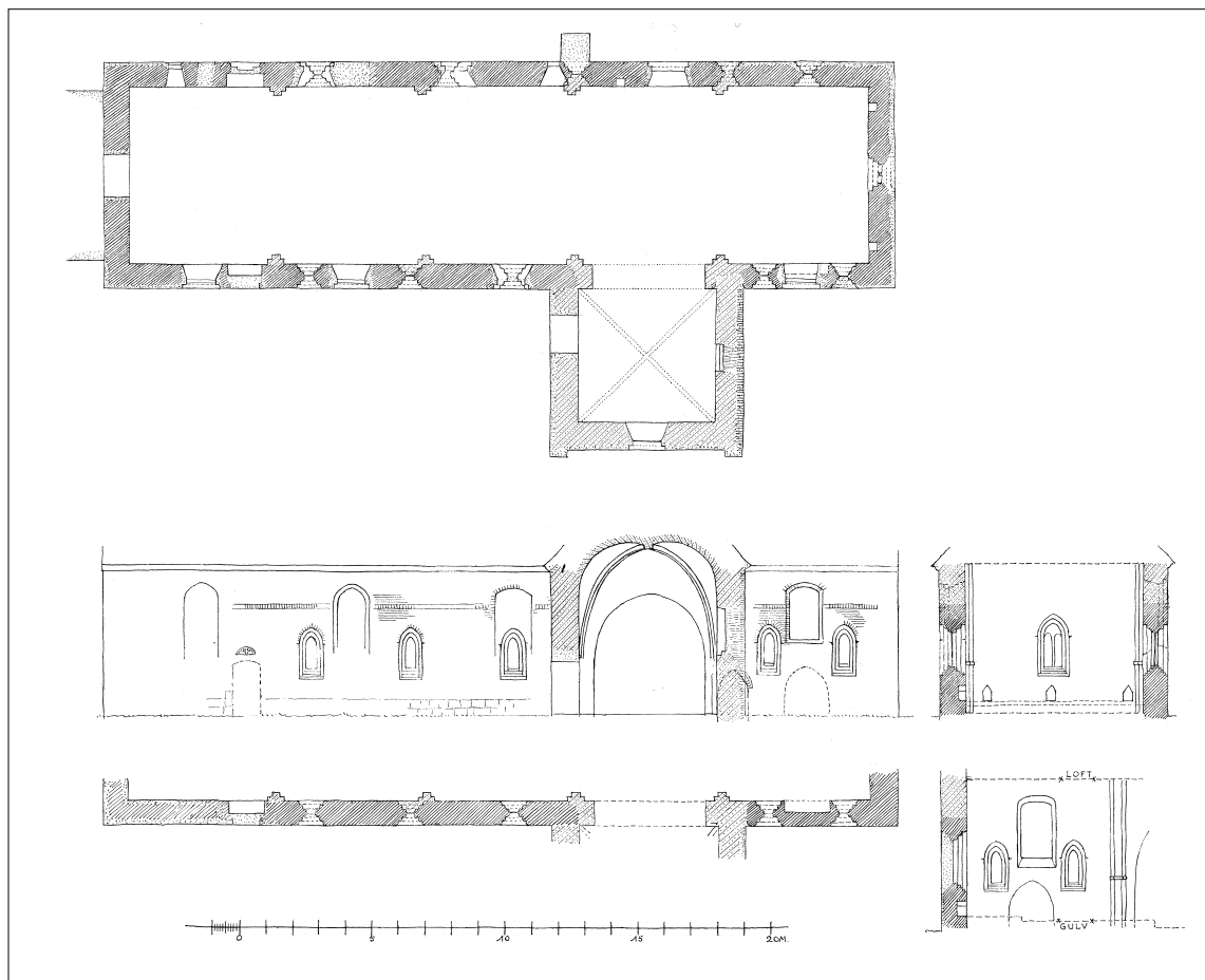
Fig. 10. Plan, snit og opstalt af sydfacaden. 1:300. Målt og tegnet af Charles Christensen 1933. – Grundriss, Schnitte und Aufriss der Südfassade.
